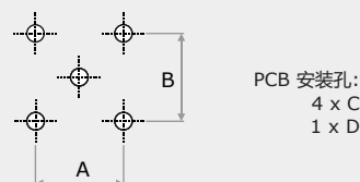
PCB板安装孔尺寸
