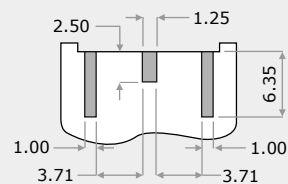
PCB板焊接建议图 ■
