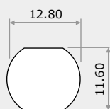
面板安装孔尺寸 ■
