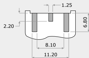
PCB板焊接建议图 ■
